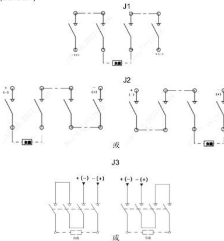
4P 外形接线图(DC1500V)
